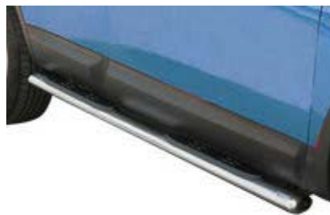
GPO/158/IX ovales Schwellerrohr mit Tritt Ø 76mm, Edelstahl
